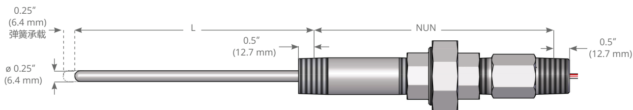
TTC 传感器
