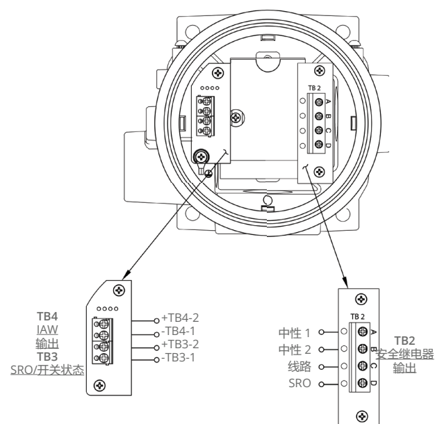
图 6: 底座外壳
