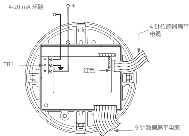
图 5: 显示模块 (背面)
