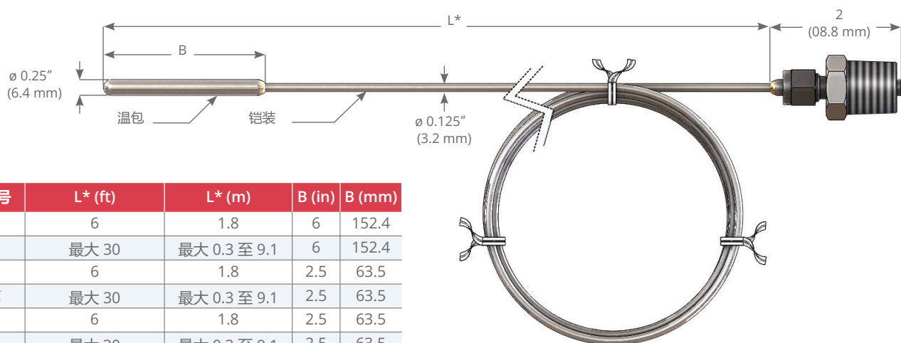
远程传感器
