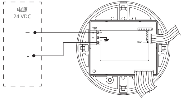
图 8：显示模块（背面）
