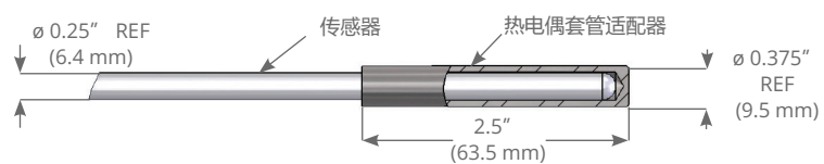
热电偶套管适配器 (选项 W081)
