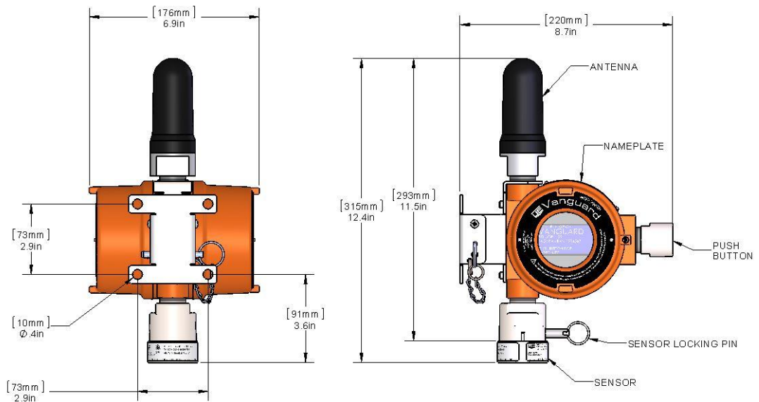
TCD60 型号的示图为标准安装
